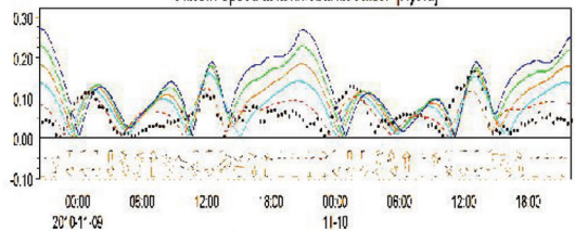
نگاره ۶- مقایسه تاریخچه زمانی سرعت‌های جزر و مدی مدل‌سازی شده به ازای اعداد مانینگ مختلف و داده‌های اندازه‌گیری در موقعیت ایستگاه کوه مبارک [هایدرا]
