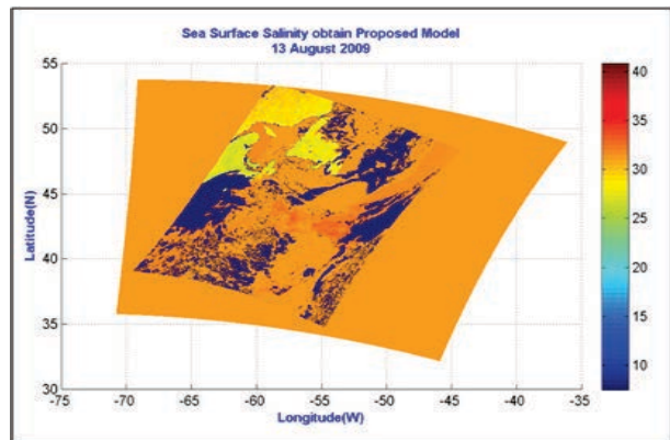
نگاره ۱۹: نقشه شوری سطحی خلیج سنت لورنس بعد از تصحیحات رادیومتریک و هندسی، در روز ۱۳ آگوست ۲۰۰۹ با استفاده از مدل پیشنهادی
