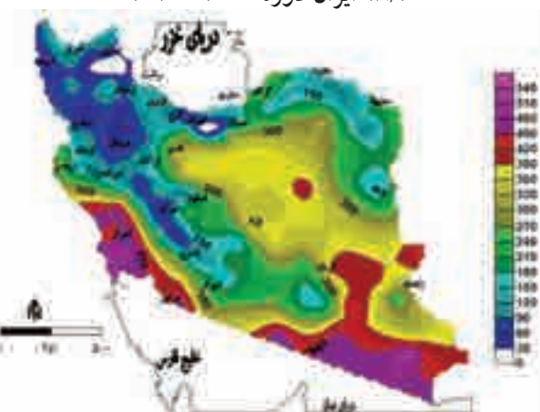
نگاره ۱۹: میانگین درجه روز سرمایش اوت آستانه دمایی ۱۸/۳ ایران دوره ۱۹۷۰-۲۰۰۴
