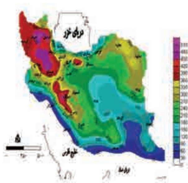
نگاره ۱: میانگین درجه روز گرمایش ژانویه آستانه دمایی ۱۱ در ایران دوره ۱۹۷۰-۲۰۰۴
