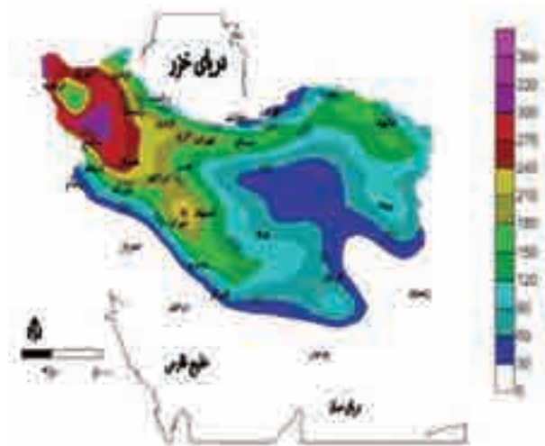
نگاره ۶: میانگین درجه روز گرمایش مارس آستانه دمایی ۱۱ در ایران در دوره ۲۰۵۰-۲۰۱۵
