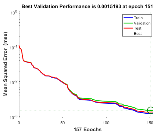
نگاره ۱۴: نمودار کارایی (خطا) شبکه عصبی بر سه مجموعه داده آموزش، ارزیابی و تست تصاویر روزانه
