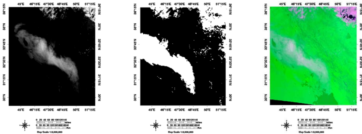
نگاره ۱۰: اعمال شاخص (۲۳-۳۱) به ترتیب از راست به چپ، ترکیب رنگی کاذب، تصویر باینری MATLAB، تصویر باینری ENVI، آستانه BTD(23-31) > 6
