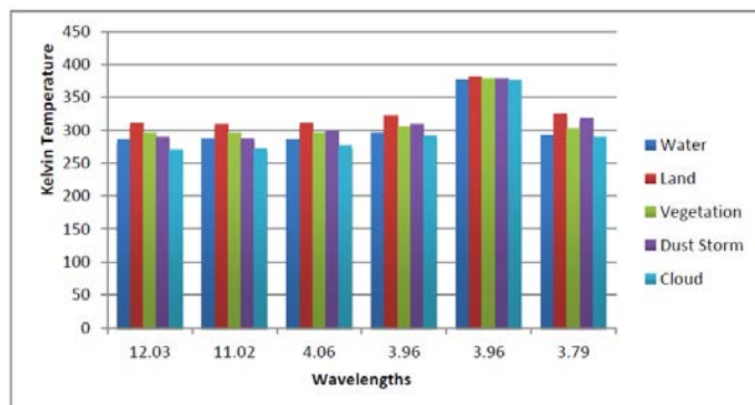
نگاره ۶: میانگین دمای روشنایی آب، زمین، گیاهان، گردوغبار، ابر برای باندهای ۲۰، ۲۱، ۲۲، ۲۳، ۳۱، ۳۲ و ۳۳ (El-Ossta, 2013:51)
