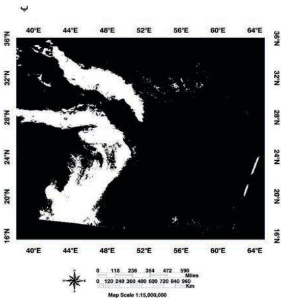
نگاره ۷: نمونه‌ای از نحوه تعیین آستانه مناسب برای بارزسازی گردوغبار: الف) BTD(31-32) < 0 (ب) BTD(31-32) < -0.5 (پ) BTD(31-32) < -1 (ت) BTD(31-32) < -1.2
