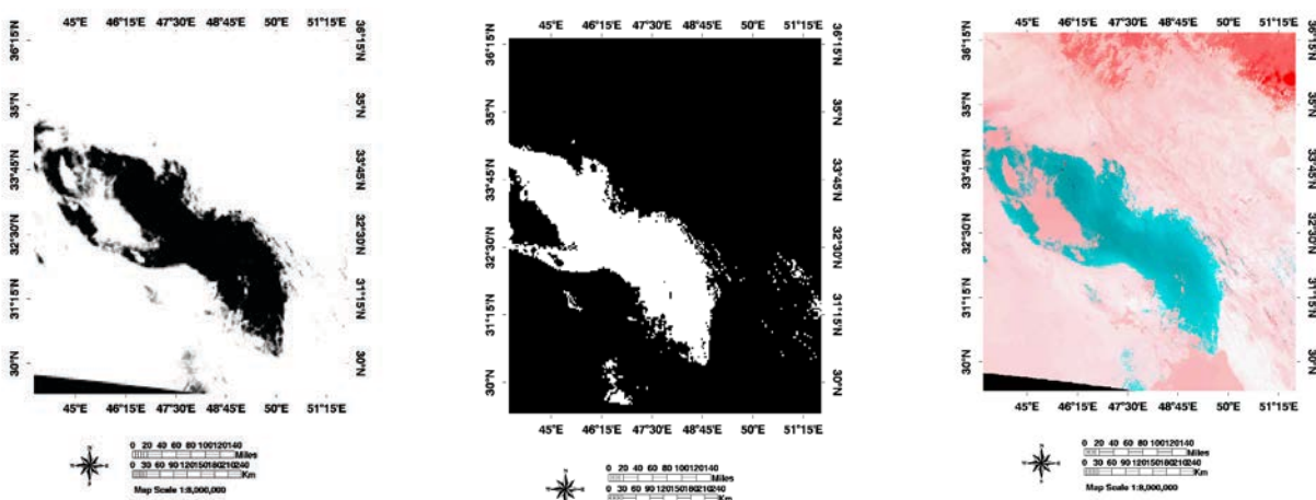
نگاره ۱۱: اعمال شاخص (۳۱-۳۲) به ترتیب از راست به چپ، ترکیب رنگی کاذب، تصویر باینری MATLAB، تصویر باینری ENVI، آستانه BTD(31-32) < (-1)
