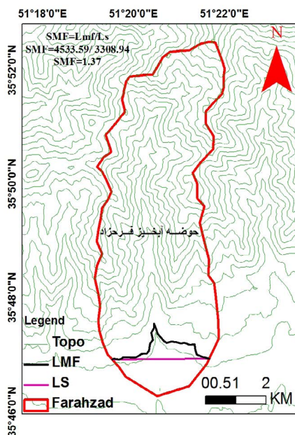
نگاره ۷: نحوه ارزیابی شاخص SMF در حوضه فرحزاد
