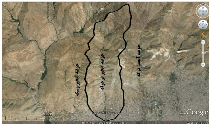
نگاره ۱. موقعیت حوضه آبخیز فرحزاد و دیگر حوضه‌های اطراف آن در شمال شهر تهران.
