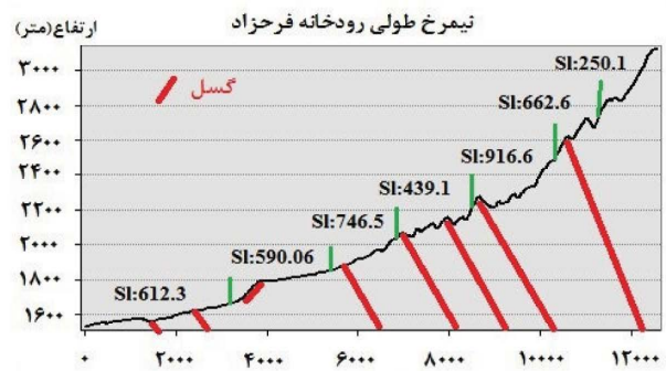
نگاره ۵: نیمرخ طولی رودخانه فرحزاد
