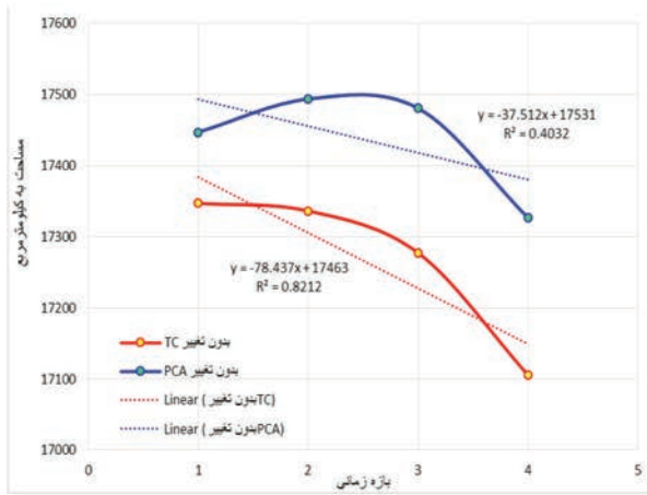
نگاره ۶: روند تغییرات PCA و TC در منطقه مورد مطالعه در طول زمان ۲۰۱۴-۱۹۷۶
