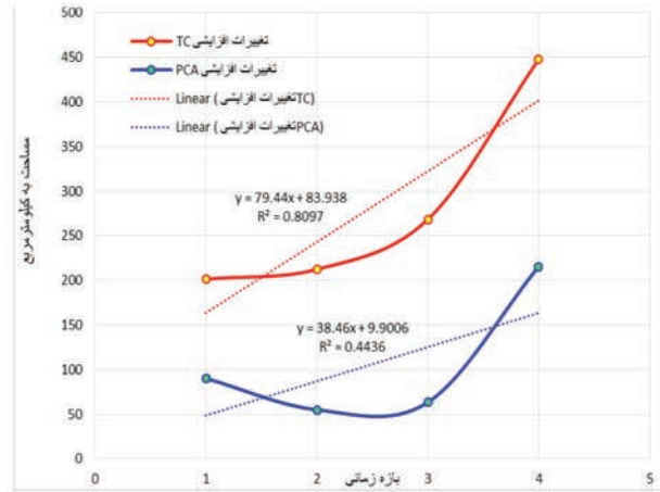
نگاره ۶: روند تغییرات PCA و TC در منطقه مورد مطالعه در طول زمان ۲۰۱۴-۱۹۷۶
