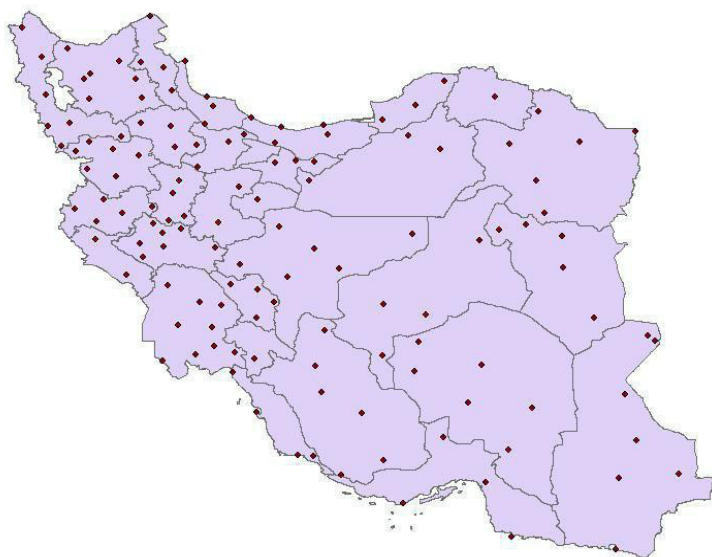
نگاره ۲: محل ایستگاه‌های سینوپتیک هواشناسی در ایران
