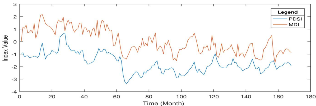
نگاره ۴: مقایسه میانگین مقادیر شاخص‌های MDI PDSI
