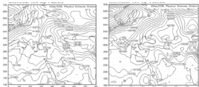
نقشه ۶- فشار دریا در ۴۸ ساعت (سمت راست) و ۲۴ ساعت (سمت چپ) قبل بارش روزهای ۱ و ۲ نوامبر ۲۰۰۰ م
