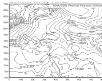
نقشه ۷ - فشار تراز دریا در روز آغاز بارش ۳ نوامبر ۲۰۰۰ م
