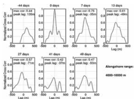
نگاره ۱۱: همبستگی‌های عرضی بین نقشه برداری منحنی میزان 2 متری خط ساحل برای 10-4 کیلومتر در ۲۰ فوریه ۲۰۰۴ و نقشه برداری‌های بعدی. روزهای بین نقشه برداری و نقشه برداری ۲۰ فوریه ۲۰۰۴، در بالای هر پلات نوشته شده است.
