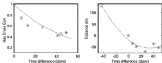
نگاره ۱۲: حداکثر همبستگی عرضی بین ۲۰ فوریه ۲۰۰۴ و نقشه برداری بعدی (*) و قبلی (0) (پانل سمت چپ)، و جابجایی حداکثر همبستگی عرضی بین نقشه برداری‌های بعدی که حرکت خط ساحل (پانل سمت راست) را برای 10-4 کیلومتر، توصیف می‌کند.
