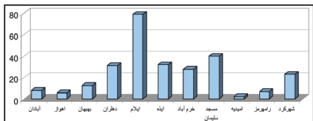
نمودار ۱: داده‌های بارش در روز ۱۱ مارس ۲۰۰۵
