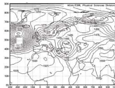
نگاره ۷: آرایش سامانه‌ها بر روی نقشه تراز ۸۵۰ هکتوپاسکال در الگوی ادغامی
