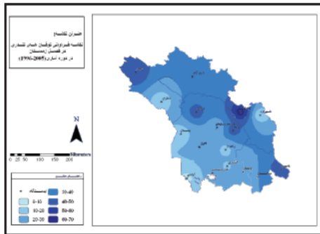
نگاره ۵: فراوانی وقوع توفان تندی در زمستان
