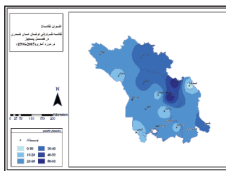
نگاره ۴: فراوانی وقوع توفان تندی در پاییز
