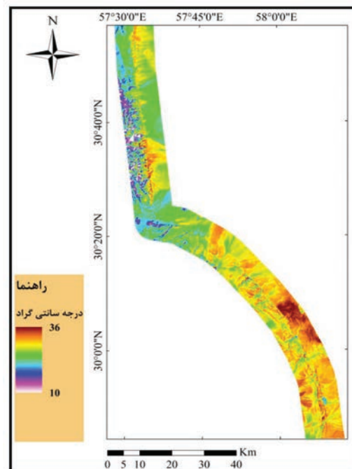
نگاره ۷: بافر ۶ كيلومتری ایجاد شده اطراف گسل‌ها در
