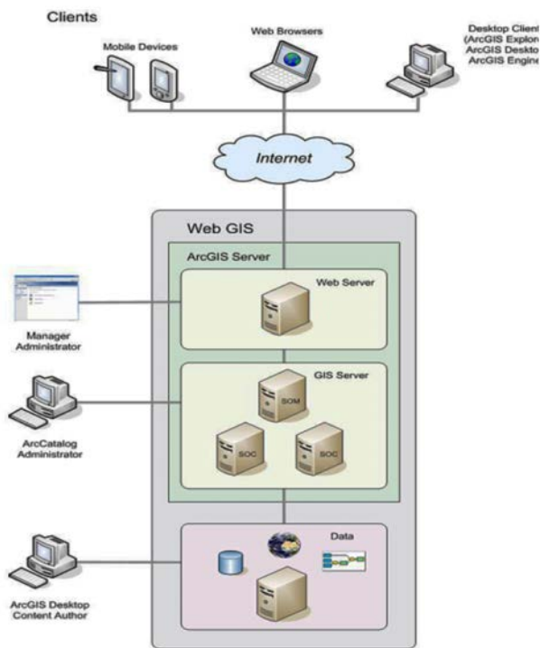
نگاره ۹: معماری نرم افزار ArcGIS-Server (Esri, 2009)
