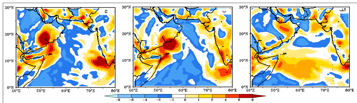
نگاره ۱۳: مقادیر تاوایی مطلق ( s^{-1} ) در زمان: شکل گیری (الف)، شدت (ب) و خاتمه (ج) چرخند حاره‌ای میکنونو
