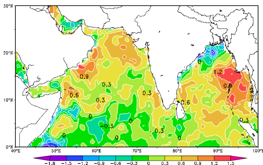
نگاره ۱۶: تغییرات ناهنجاری‌های ایجاد شده در مؤلفه‌ی SST طی دوره‌ی فعالیت چرخندهای حاره‌ای ساگار و میکونو نسبت به شرایط نرمال اقلیمی (۱۹۸۰-۲۰۱۵)
