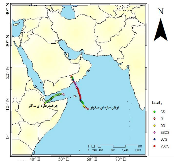
نگاره ۱: موقعیت شکل‌گیری چرخندهای مورد مطالعه در دریای عرب
