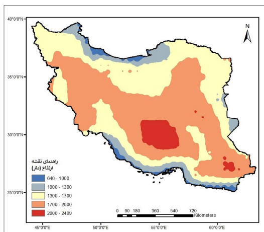
نگاره ۱۲: نقشه ارتفاع لایه مرزی ماه جون (۱۹۰۹-۲۰۲۱)
