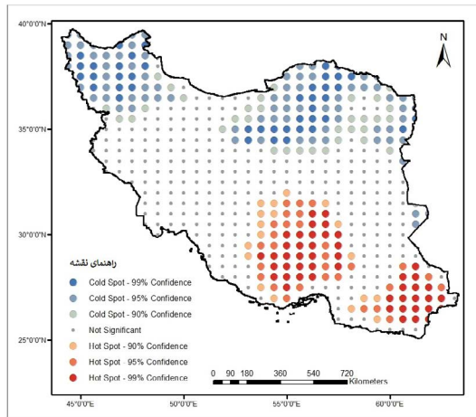
نگاره ۲۳: نقشه مدل Getis Ord ماه نوامبر (۱۹۵۹-۲۰۲۱)
