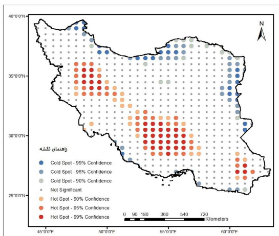
نگاره ۱۹: نقشه مدل Getis Ord ماه سپتامبر (۲۰۲۱-۱۹۵۹)
