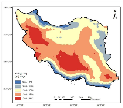
نگاره ۱۶: نقشه ارتفاع لایه مرزی ماه آگوست (۱۹۵۹-۲۰۲۱)
