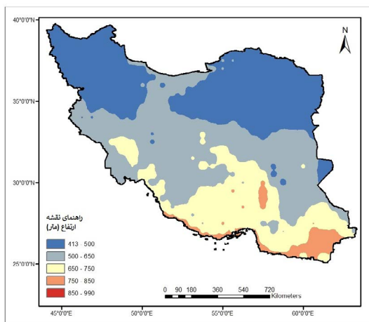
نگاره ۲۴: نقشه ارتفاع لایه مرزی ماه دسامبر (۱۹۵۹-۲۰۲۱)
