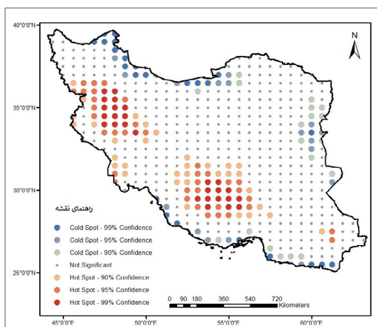
نگاره ۱۷: نقشه مدل Getis Ord ماه آگوست (۱۹۵۹-۲۰۲۱)
