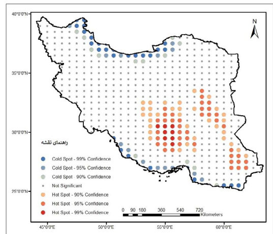
نگاره ۱۱: نقشه مدل Getis Ord ماه می (۱۹۰۹-۲۰۲۱)
