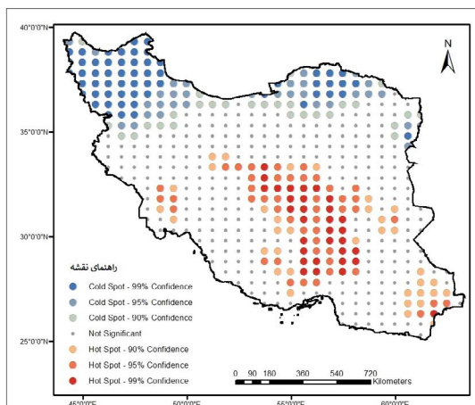
نگاره ۵: نقشه مدل Getis Ord ماه فوریه (۱۹۵۹-۲۰۲۱)
