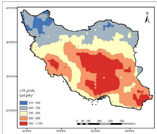
نگاره ۴: نقشه ارتفاع لایه مرزی ماه فوریه (۱۹۵۹-۲۰۲۱)
