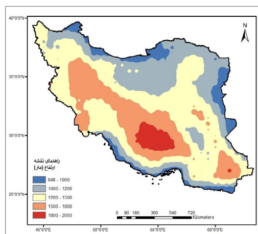
نگاره ۱۸: نقشه ارتفاع لایه مرزی ماه سپتامبر (۲۰۲۱-۱۹۵۹)
