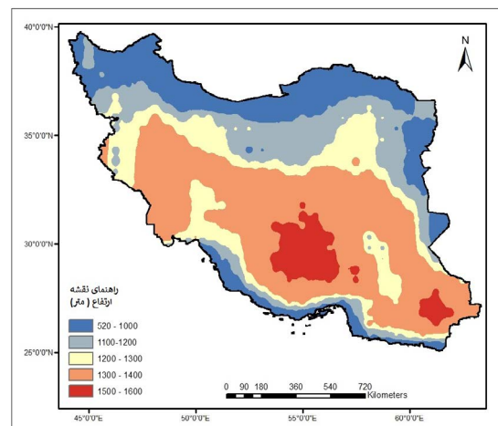
نگاره ۲۶: نقشه میانگین ارتفاع لایه مرزی سالانه (۱۹۵۹-۲۰۲۱)
