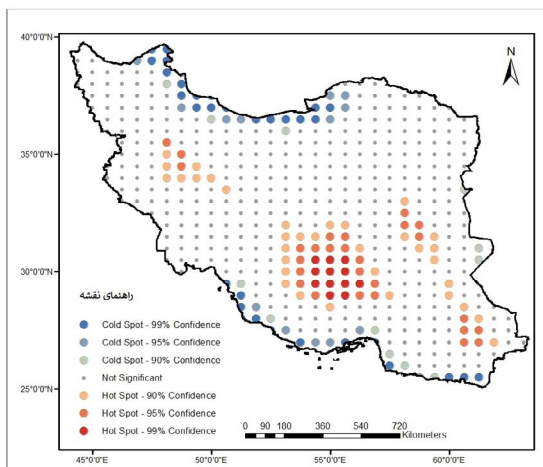
نگاره ۱۳: نقشه مدل Getis Ord ماه جون (۱۹۰۹-۲۰۲۱)
