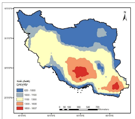
نگاره ۲۰: نقشه ارتفاع لایه مرزی ماه اکتبر (۲۰۲۱-۱۹۵۹)
