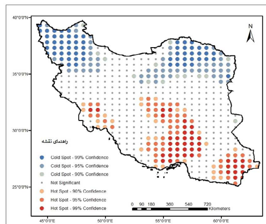
نگاره ۳: نقشه مدل Getis Ord ماه ژانویه (۱۹۵۹-۲۰۲۱)
