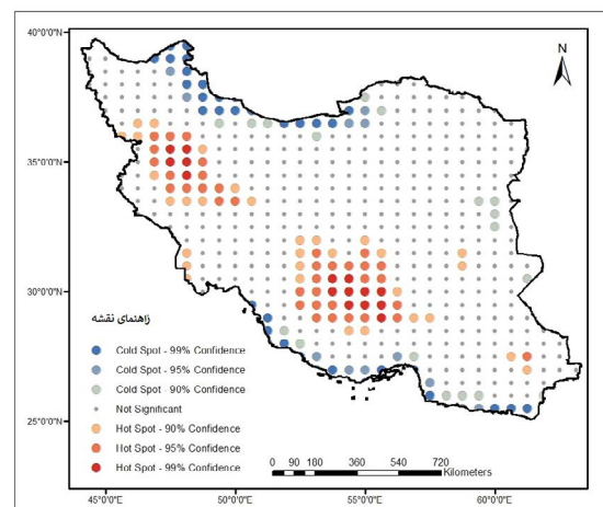
نگاره ۱۵: نقشه مدل Getis Ord ماه جولای (۱۹۵۹-۲۰۲۱)
