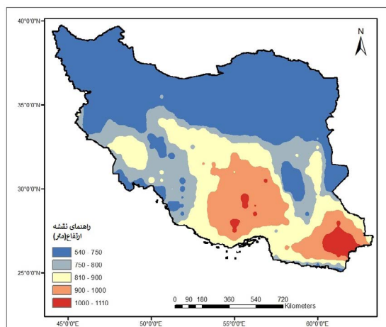
نگاره ۲۲: نقشه ارتفاع لایه مرزی ماه نوامبر (۱۹۵۹-۲۰۲۱)
