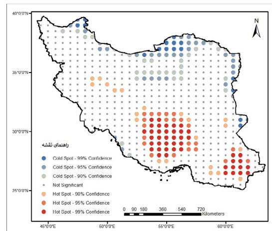
نگاره ۲۱: نقشه مدل Getis Ord ماه اکتبر (۱۹۵۹-۲۰۲۱)
