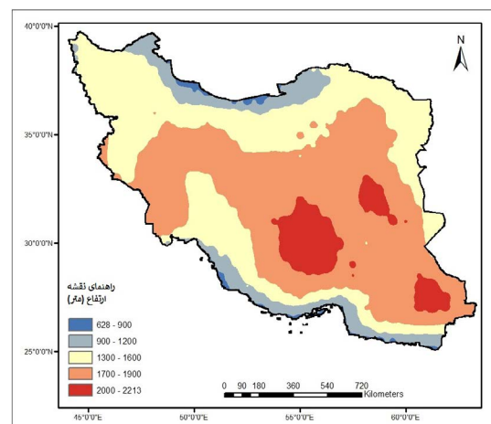
نگاره ۱۰: نقشه ارتفاع لایه مرزی ماه می (۱۹۰۹-۲۰۲۱)
