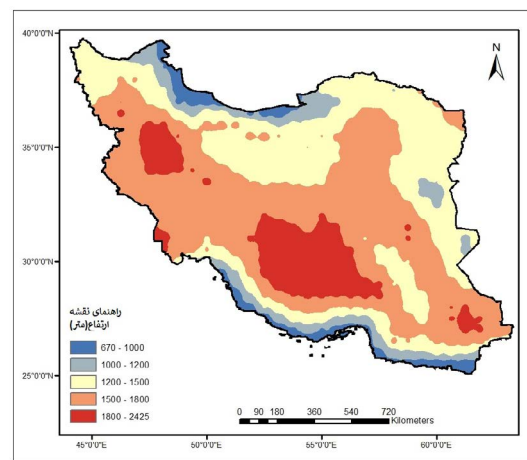
نگاره ۱۴: نقشه ارتفاع لایه مرزی ماه جولای (۱۹۵۹-۲۰۲۱)
