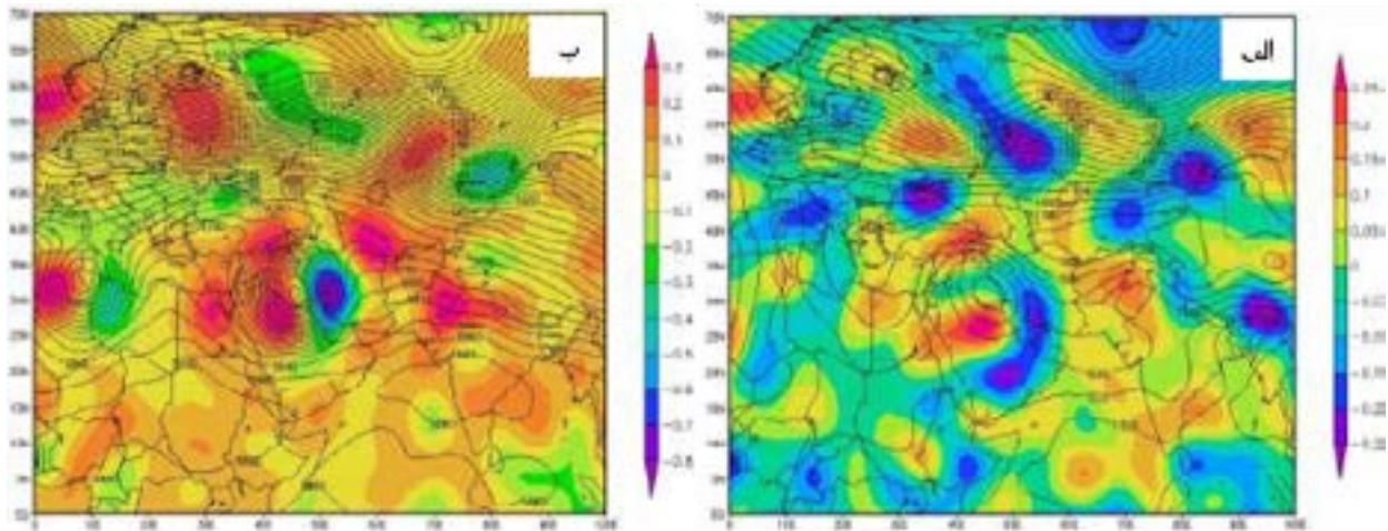
نگاره ۲: الف- نقشه ارتفاع ژئوپتانسیل و امگای تراز ۸۵۰ هکتوپاسکال ب- نقشه ارتفاع ژئوپتانسیل و امگای تراز ۵۰۰ هکتوپاسکال در روز بارشی ۲۷ دی ماه ۱۳۷۴
