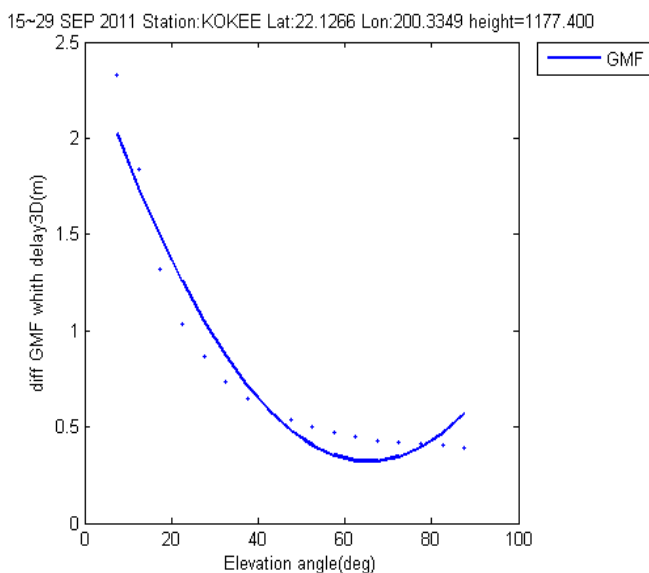
نگاره ۴: ایستگاه KOKEE در بازه زمانی ۱۵ الی ۲۹ سپتامبر سال ۲۰۱۱ میلادی، اختلاف ردیابی اشعه سه بعدی با توابع نگاشت GMF نسبت به زاویه ارتفاعی
