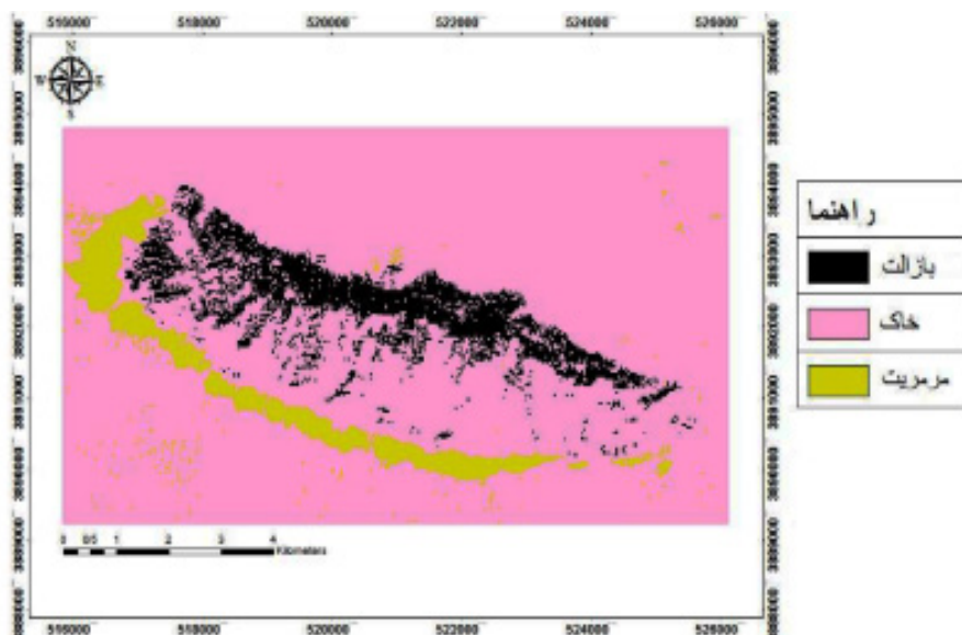
نگاره ۱۱: نمایی از نقشه تهیه شده از منطقه با ۳ طبقه بندی بازالت، خاک و مرمیریت
