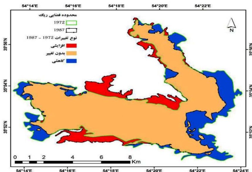
نگاره ۵: پویایی و تغییرات رفتاری ریگ غربی کویر دامغان در بازه ۱۹۷۲ تا ۱۹۸۷
