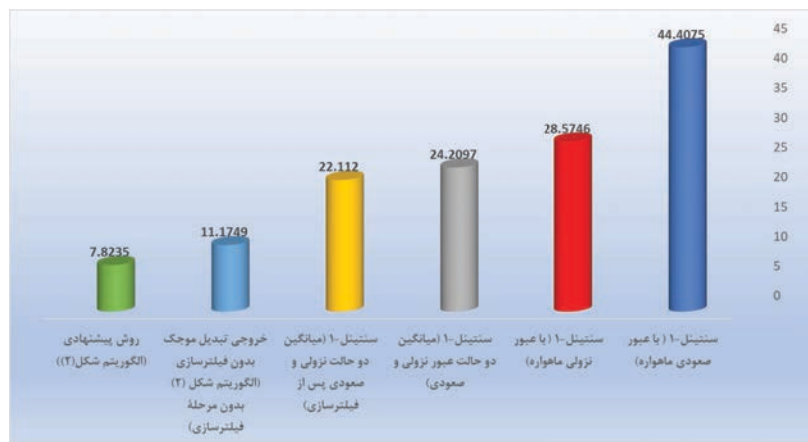
نگاره ۸: مقایسه دقت DEMهای به دست آمده از روش های مختلف براساس معیار RMSE (متر)
