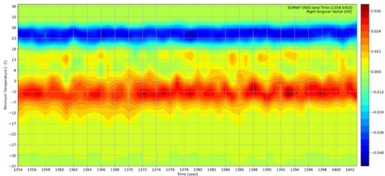
نگاره ۷: نمرات مؤلفه اول
