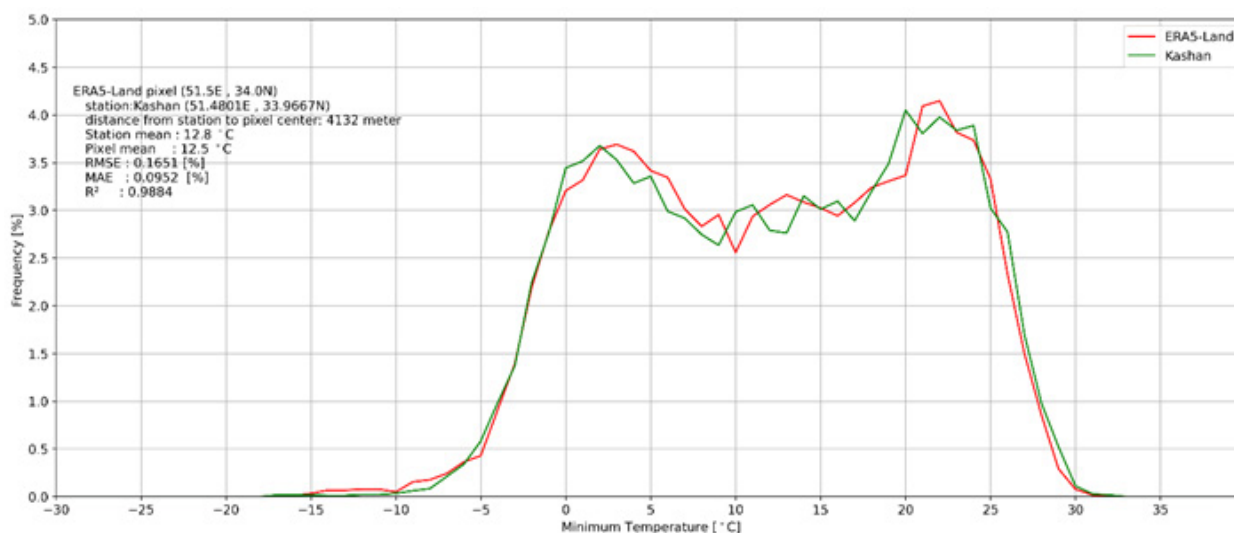
نگاره ۳: مقایسه توزیع فراوانی دمای کمینه ایستگاه کاشان با داده‌های بازکاوی
