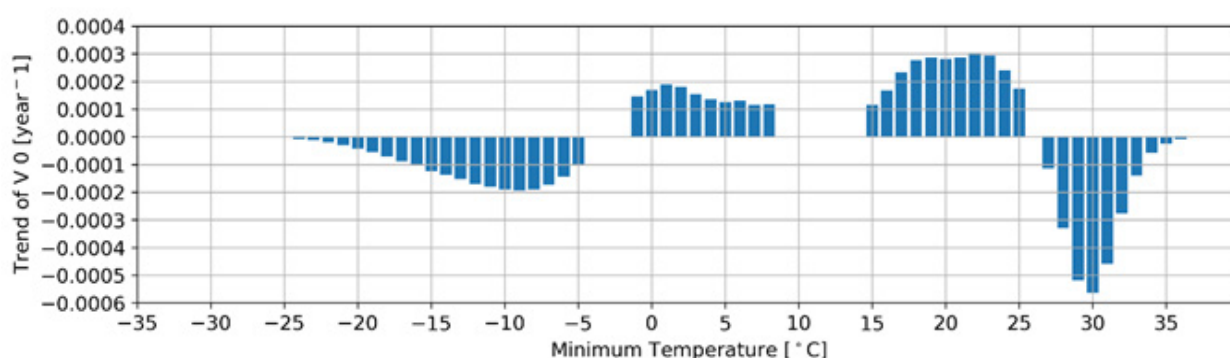
نگاره ۱۰: روند بردار ویژه نخست
