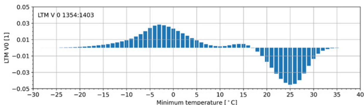
نگاره ۸: میانگین بلندمدت بردار ویژه نخست
