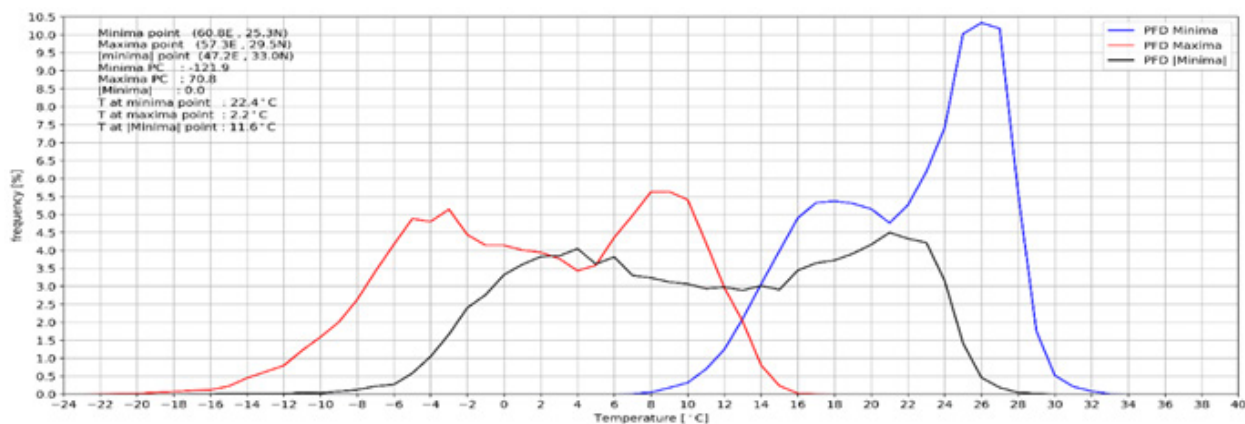
نگاره ۹: توزیع فراوانی دمای کمینه بر روی نقاطی با کمترین (آبی)، بیشترین (سرخ) و نمره مؤلفه صفر (سیاه)
