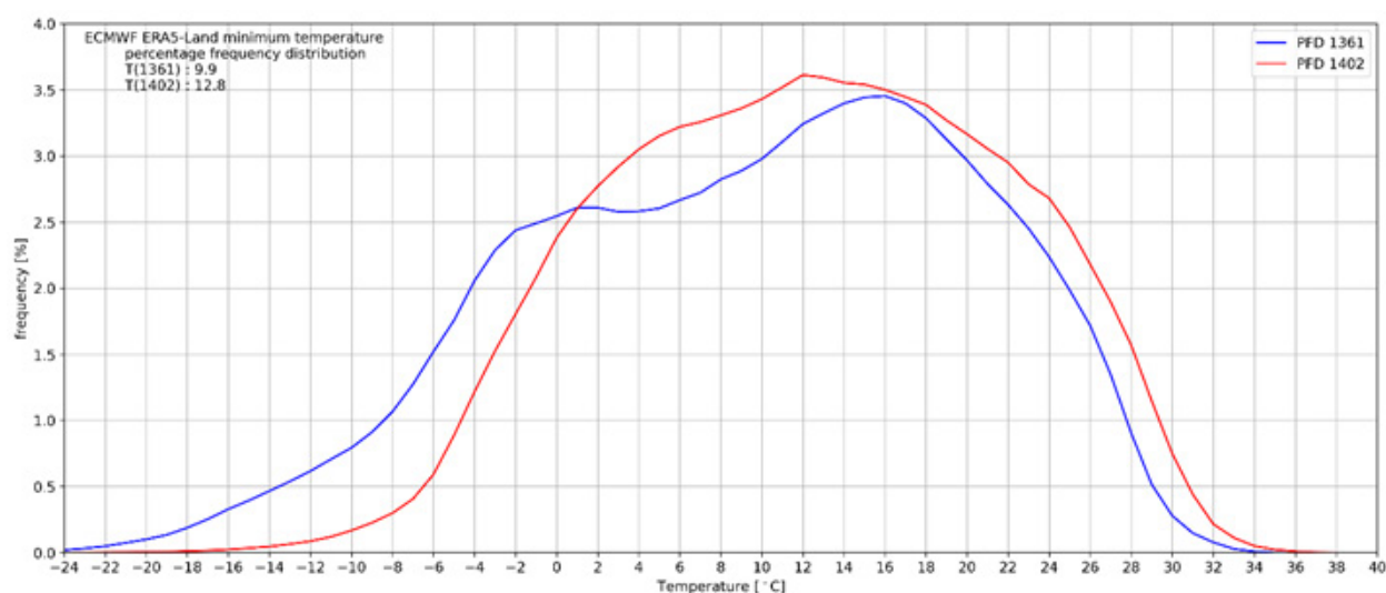
نگاره ۵: میانگین وزنی مکانی (بر روی ایران) توزیع فراوانی دمای کمینه در سال‌های ۱۳۶۱ و ۱۴۰۲
