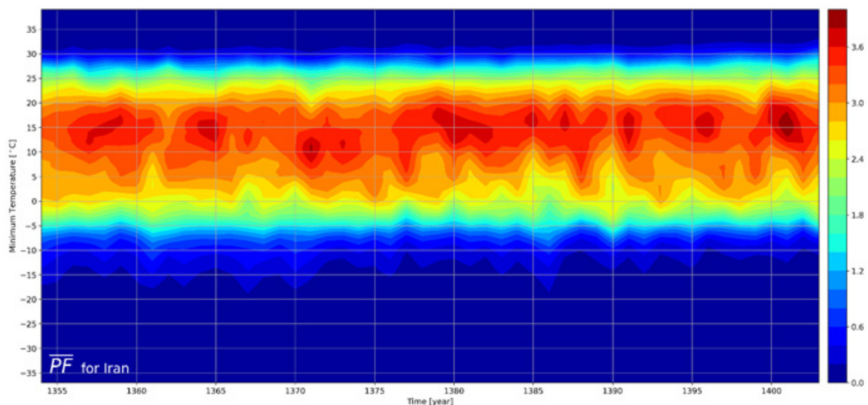
نگاره ۴: سری زمانی (۱۴۰۳-۱۳۵۴) میانگین وزنی مکانی (بر روی ایران) توزیع فراوانی دمای کمینه
