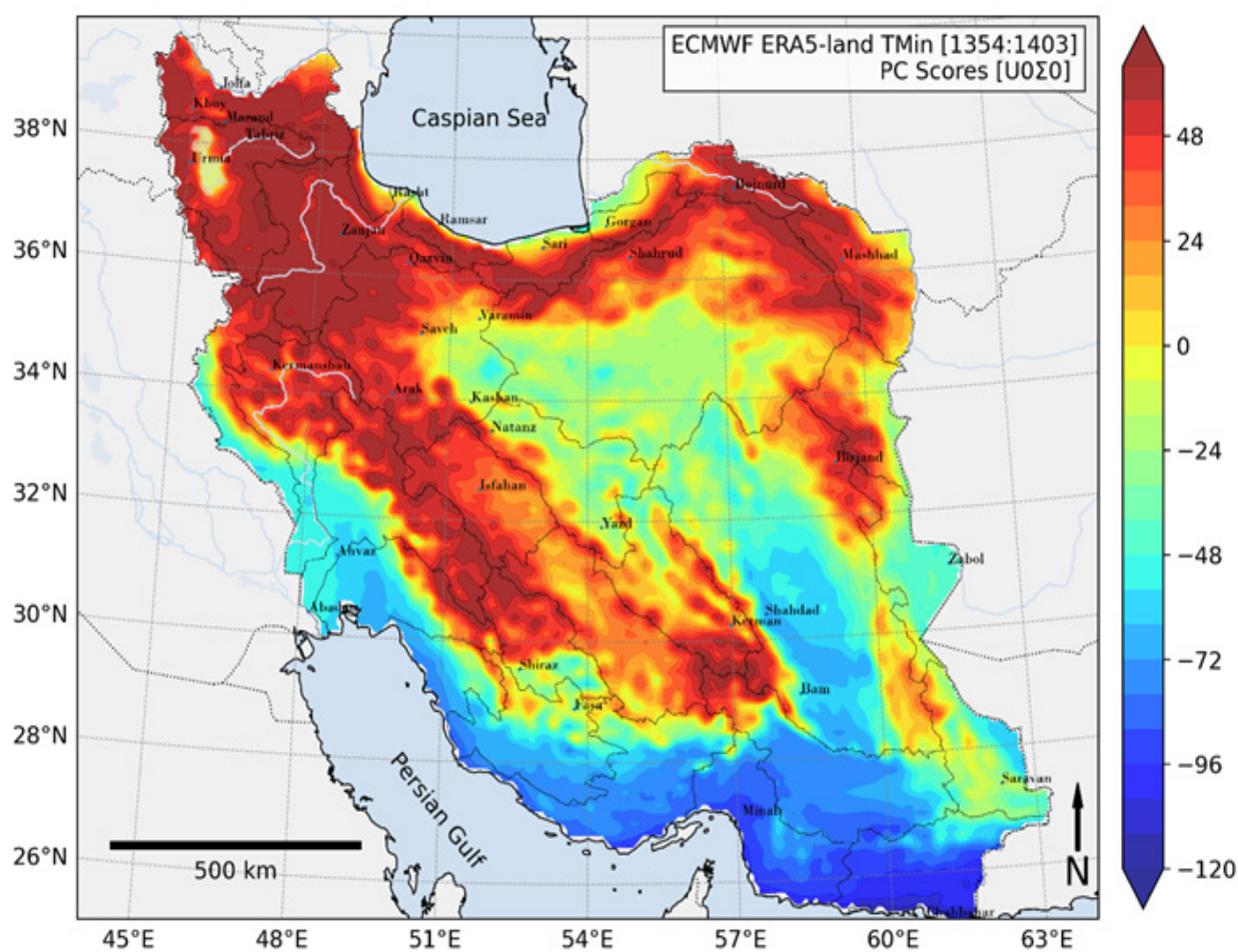
نگاره ۶: نمرات مؤلفه اول
