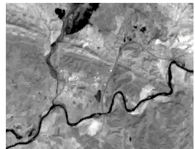
نگاره ۱۱: باند ۸ تصویر ماهواره ستینل
