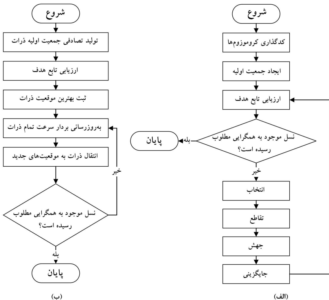
نگاره ۱: الف) فلوچارت مراحل پیاده‌سازی الگوریتم ژنتیک (Saeidian et al, 2016) ب) فلوچارت مراحل پیاده‌سازی الگوریتم ازدحام ذرات (پیاده‌کومسوار و همکاران، ۱۳۹۸)
