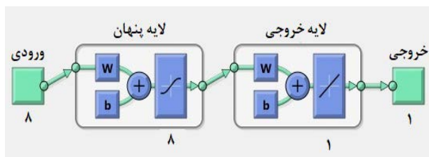
نگاره ۷: معماری شبکه عصبی حاصل از متغیرهای منتخب رویکرد پیش‌رونده به منظور شبیه‌سازی دمای بیشینه ایستگاه همدید یزد در دوره آماری ۲۰۹۵-۲۰۰۶
