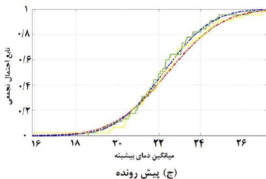
نگاره ۵: تابع احتمال تجمعی و برازش منحنی بر میانگین بیشینه دمای ماه اکتبر ایستگاه همدید یزد و مقادیر برآورد شده براساس انتخاب متغیرهای توضیحی با رویکردهای مختلف برای دوره آماری ۱۹۶۱-۲۰۰۵
